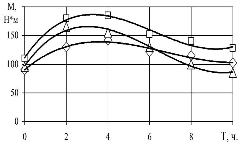
Рисунок 1 Изменение момента трения при износных испытаниях образцов: ◇ - из чугуна, □ - из стали 45, Δ - с покрытием из стали 40
