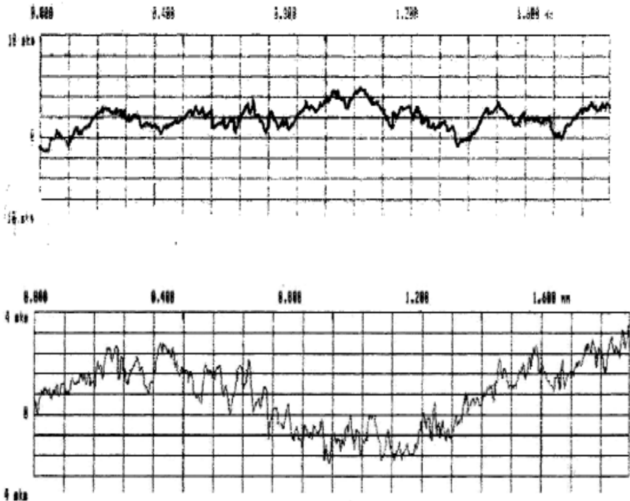
Рисунок 2 Профилограммы образцов до и после износных испытаний Вестник БГАУ / Vestnik BSAU, 2010, №1
