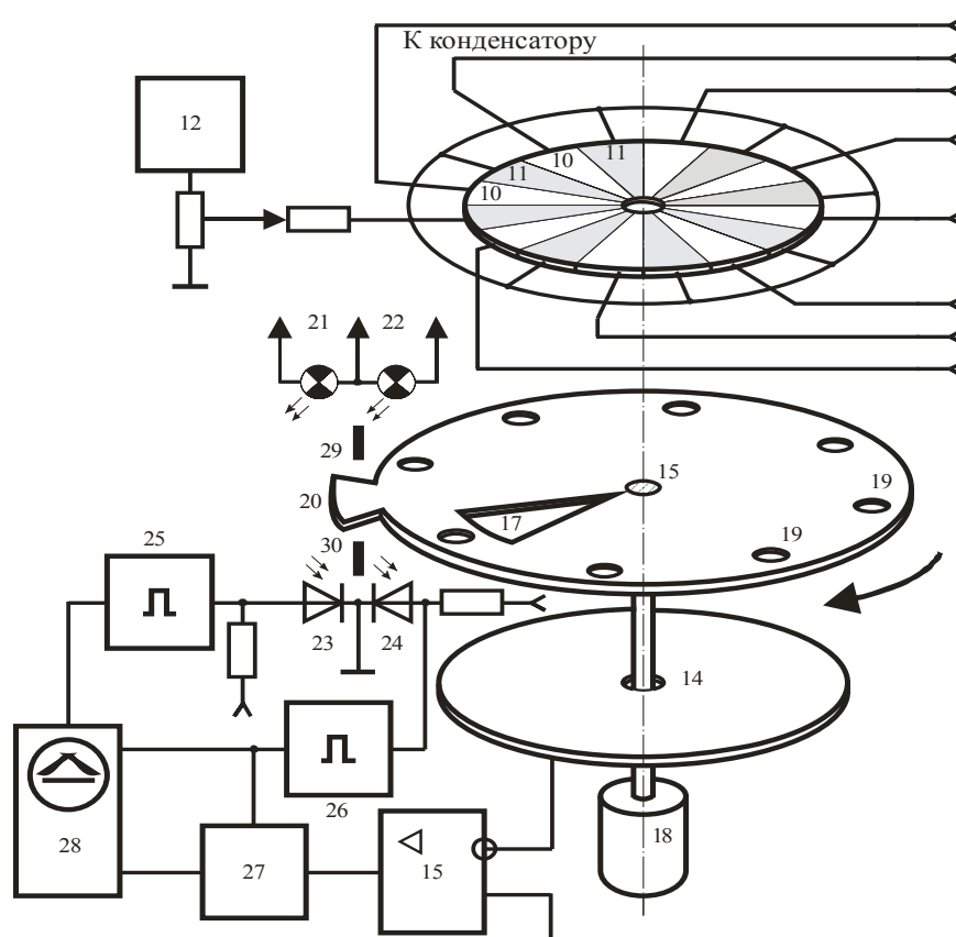
Рисунок 2 Схема емкостного коммутатора и измерительного блока анализатора электрических подвижностей аэрозолей
